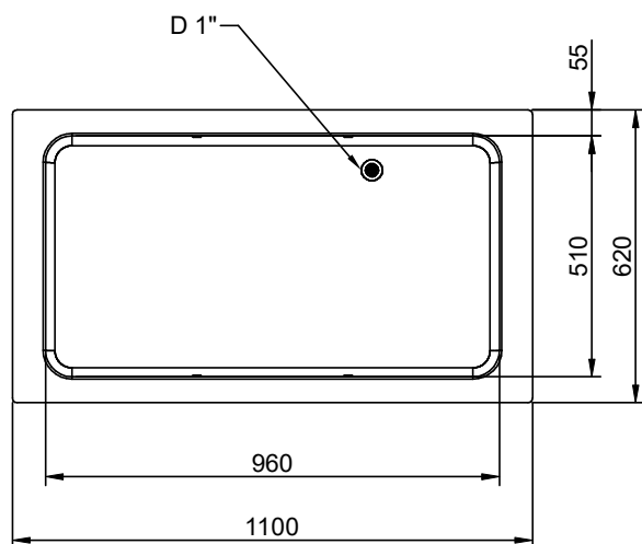
Boven aanzicht
