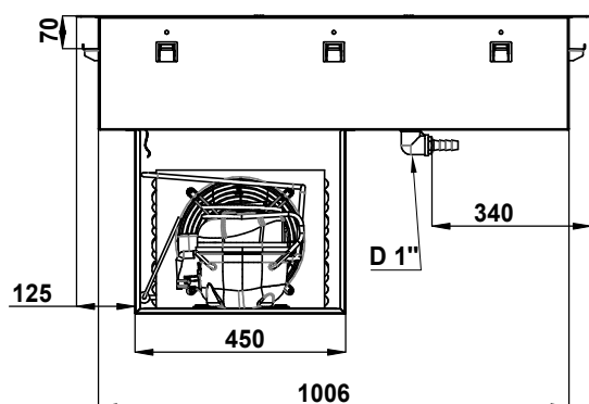
Zij aanzicht
